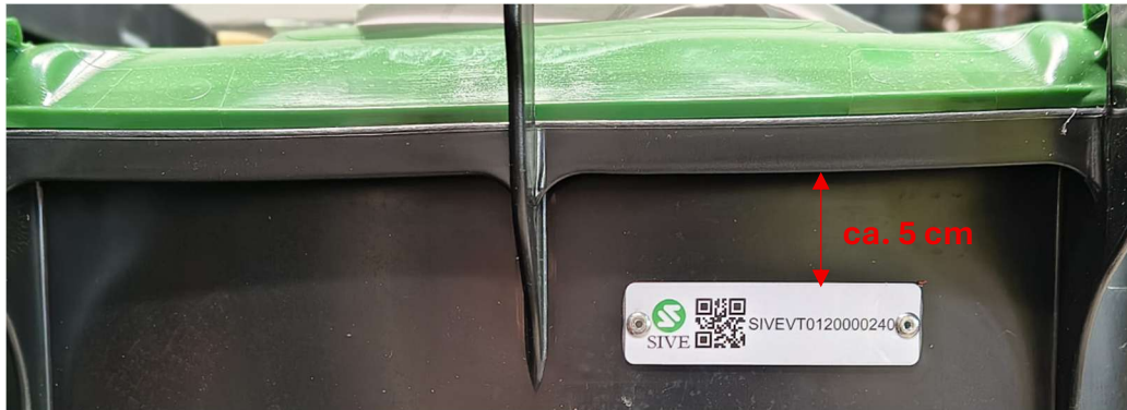
Foto 1: Posizione Tag-RFID in contenitore con 3 (o meno) nervature di rinforzo Tag-RFID da rivettare sul lato destro, in zona centrale, a ca. 5 cm dal bordo superiore del fusto
