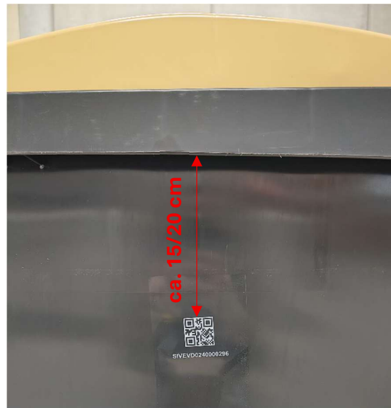
Foto 3: Posizione stampa laterale
